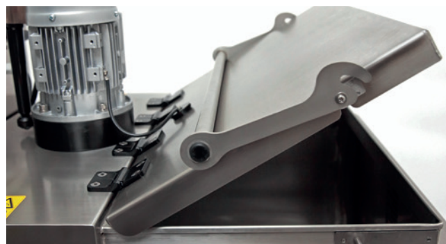
Tankdeckel mit Easy-Stop Scharnieren
